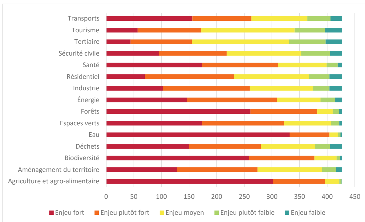
Figure 78 : Le niveau d'importance des enjeux face au changement climatique
